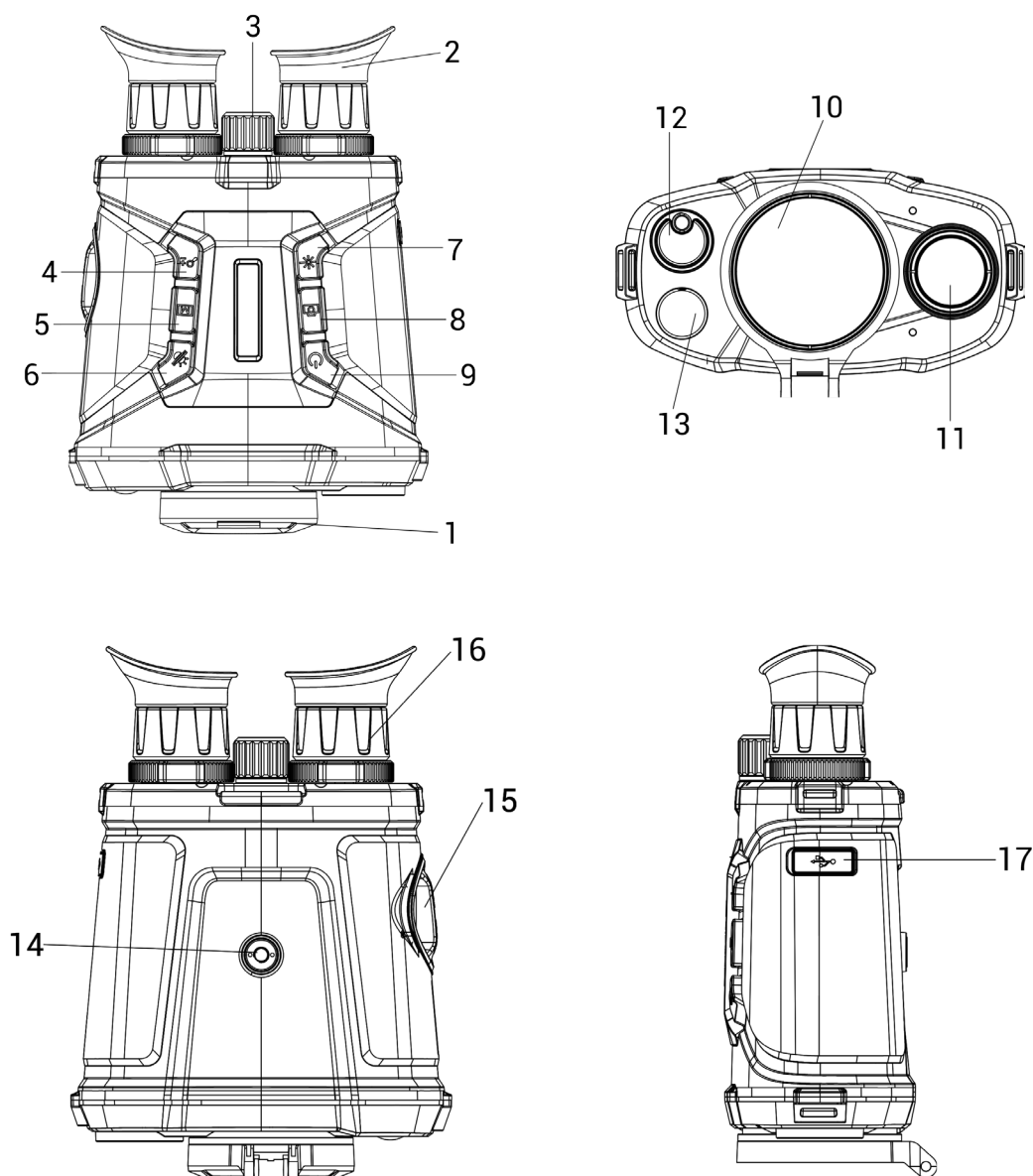
Figur 1-1 Enhetens utseende
